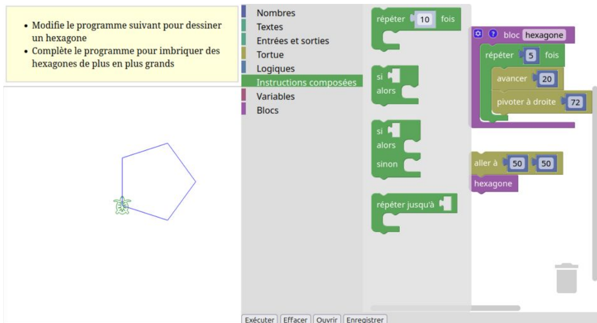
Figure 3: Une tâche de découverte des paramètres des blocs en 3 e
