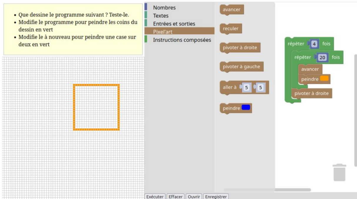
Figure 2: Une tâche de découverte de l'imbrication de boucles bornées en 5 e
